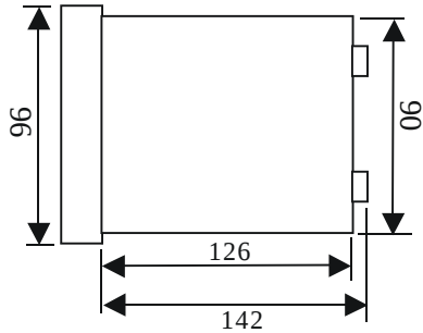
侧视图
